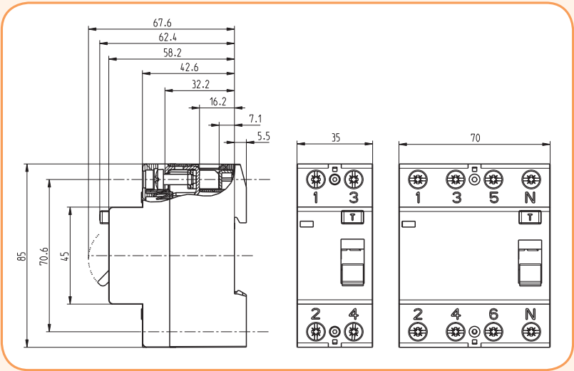
EFI 100A
