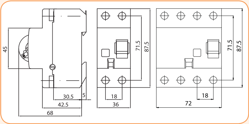
EFI 16-80A
